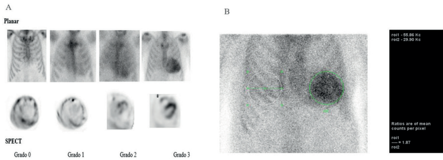
Fig. 4. A) Ejemplo de análisis semicuantitativo de la captación de 99m Tc-HMDP en imágenes planares y de SPECT. B) Análisis cuantitativo con resultado de la relación H/CL = 1,87.
